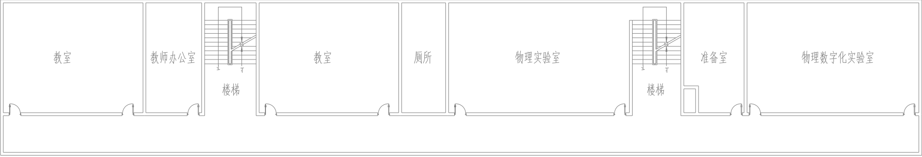
雄州初级中学2#教学楼二层平面图
