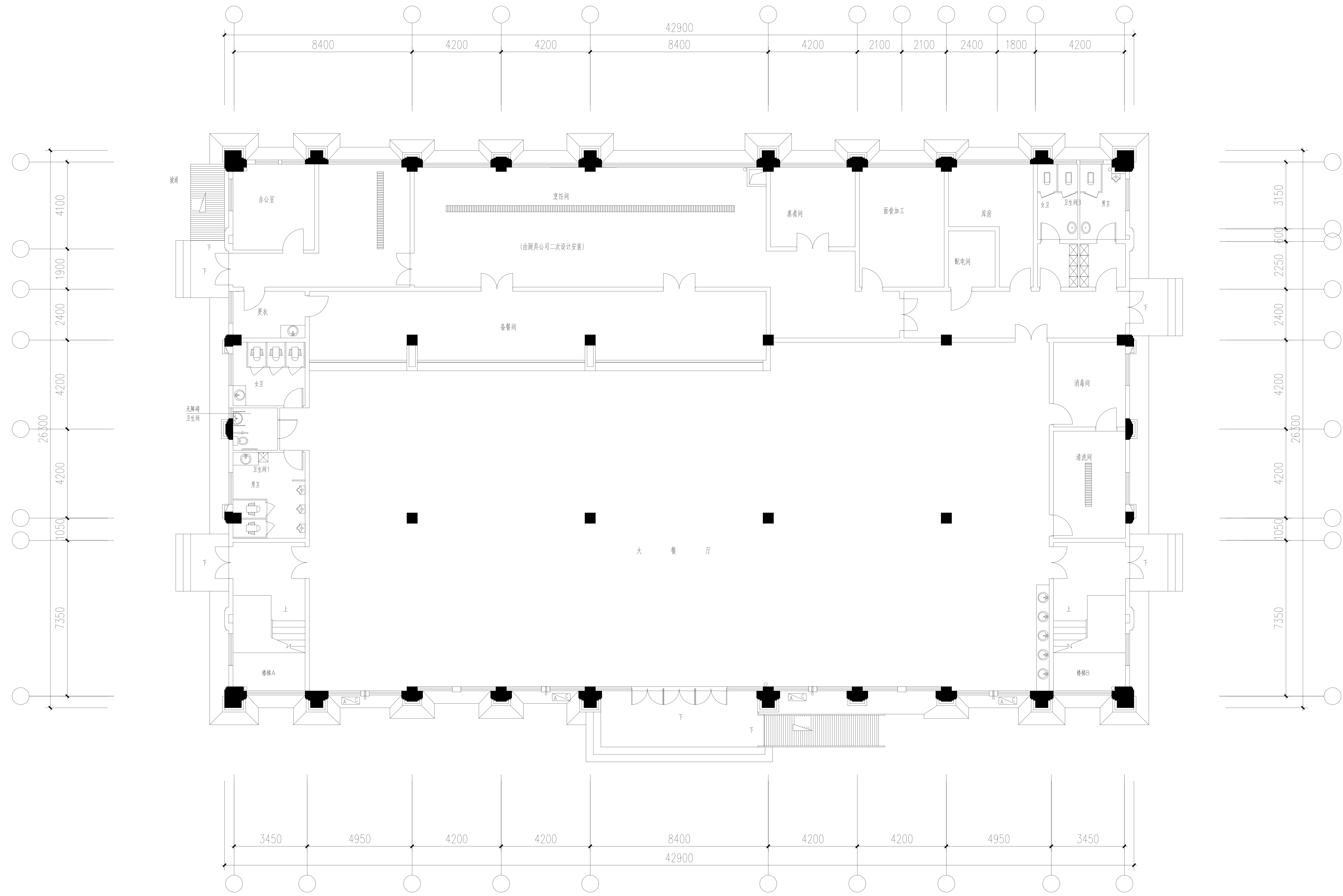
食堂及风雨操场一层平面图
