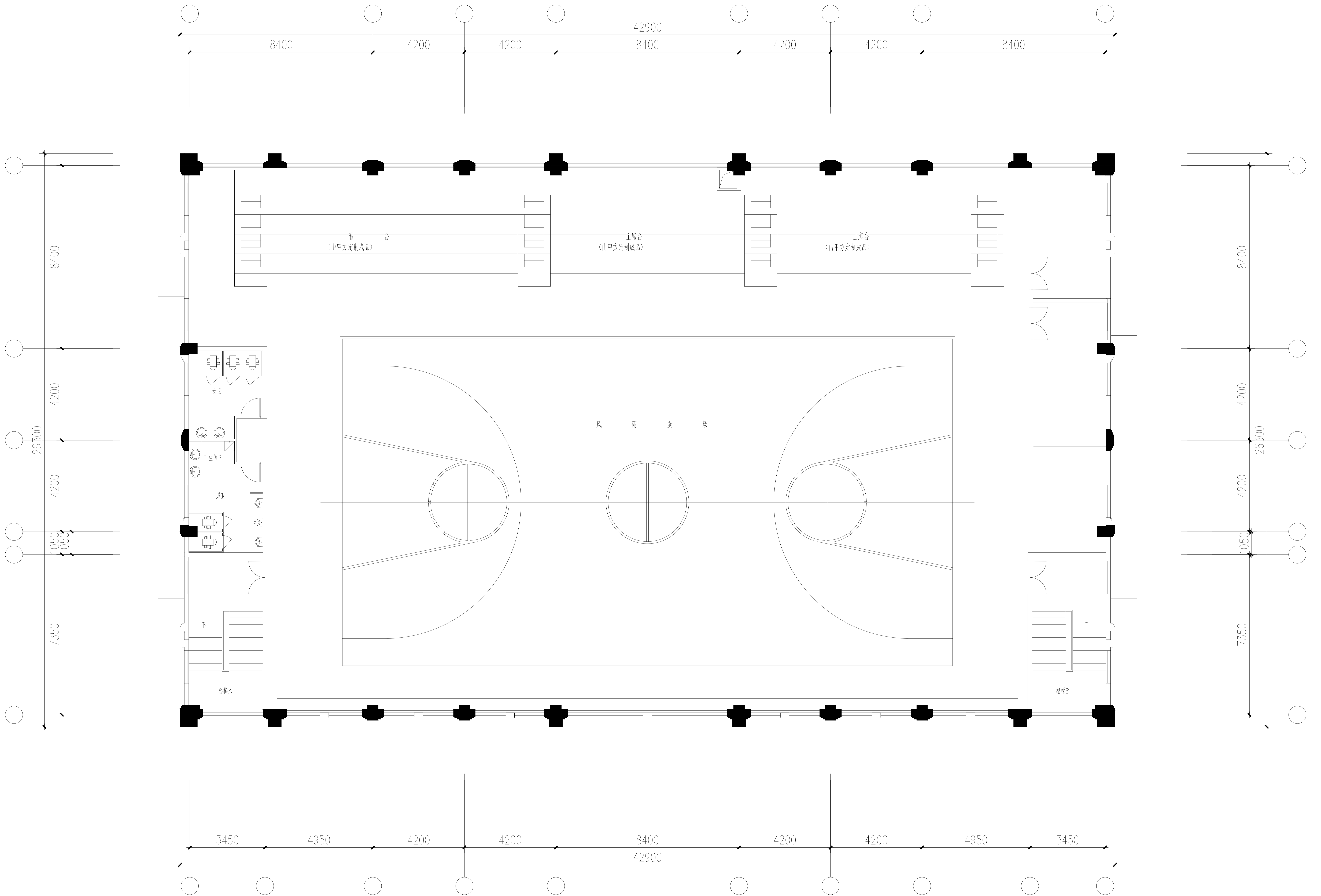
食堂及风雨操场二层平面图
