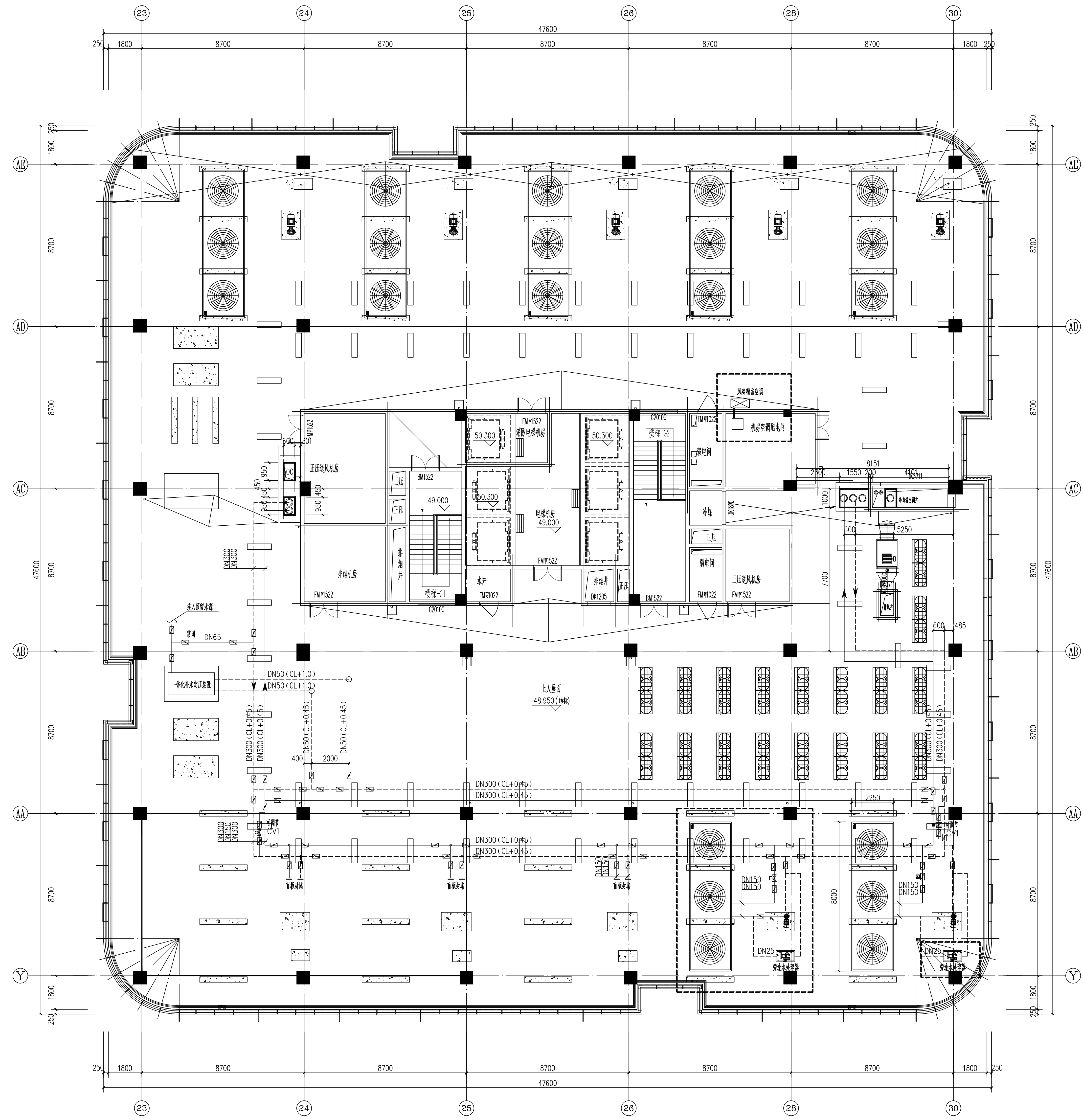
十层顶空调水系统平面图
