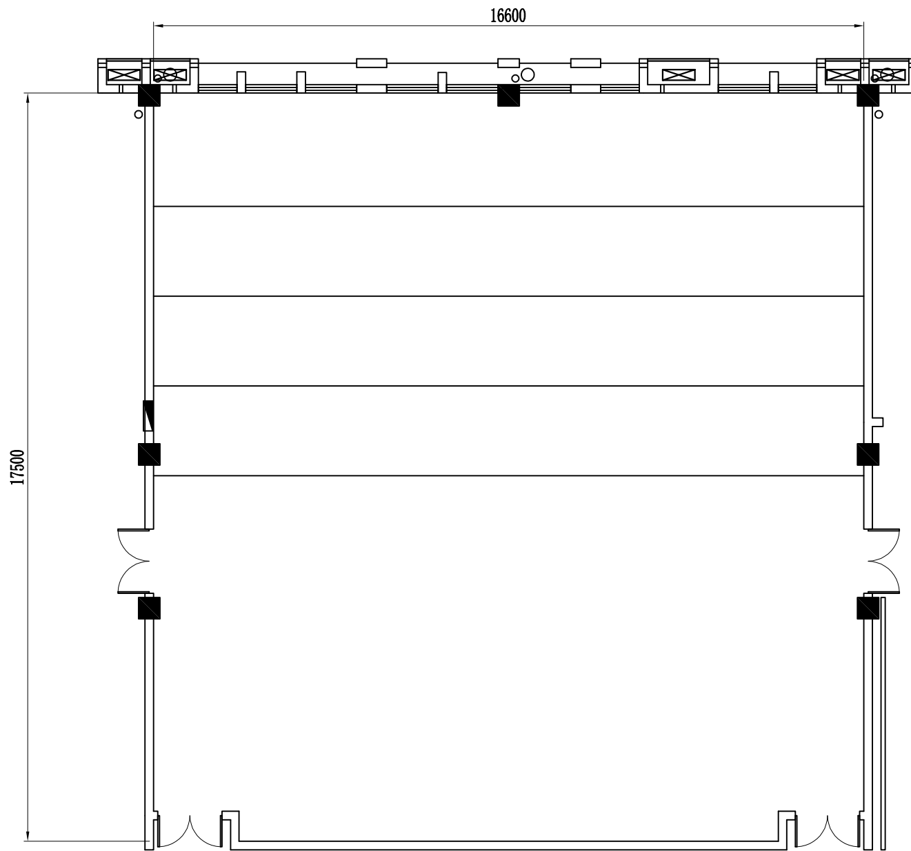
合班礼堂平面图
