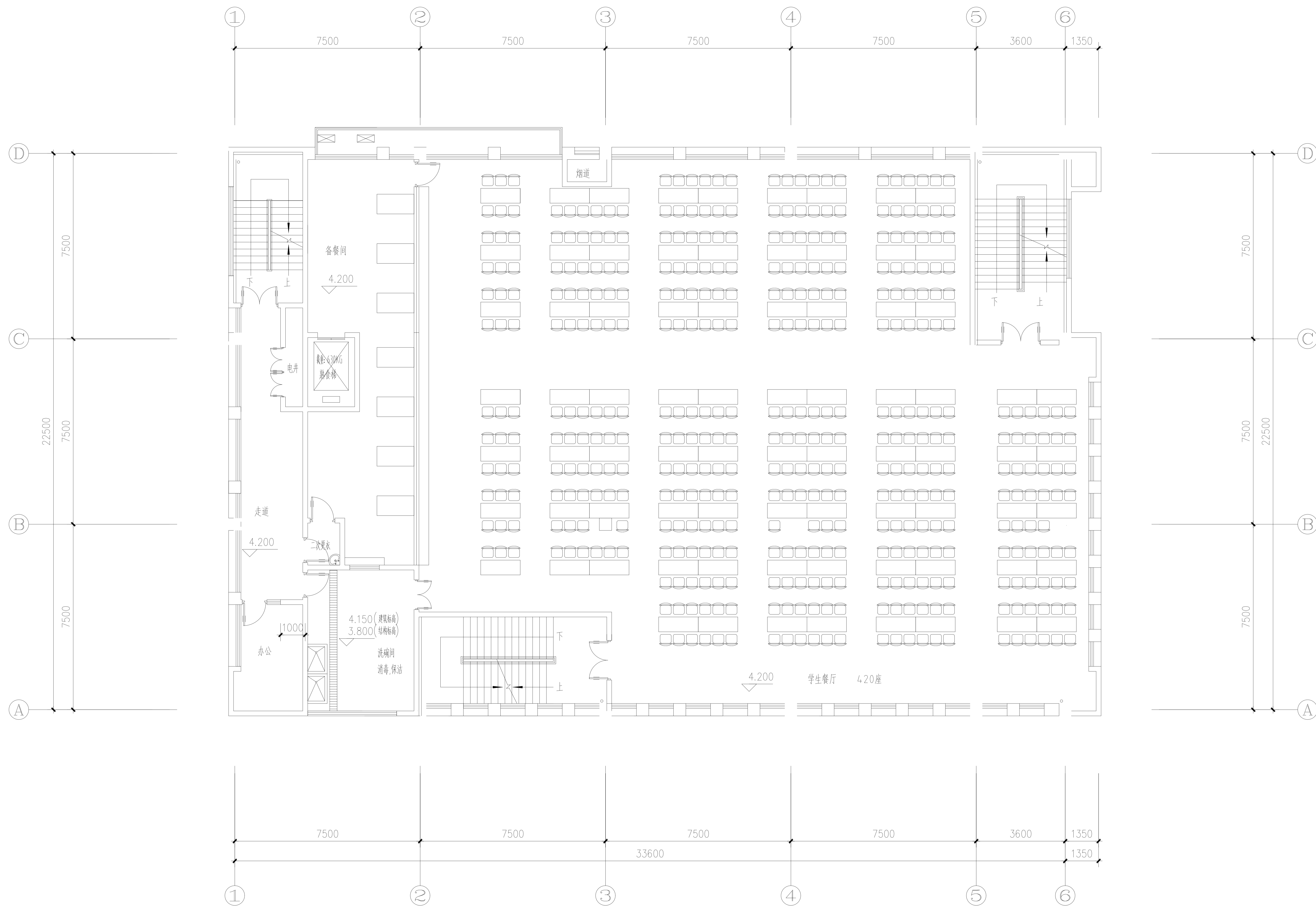
食堂二层平面图
