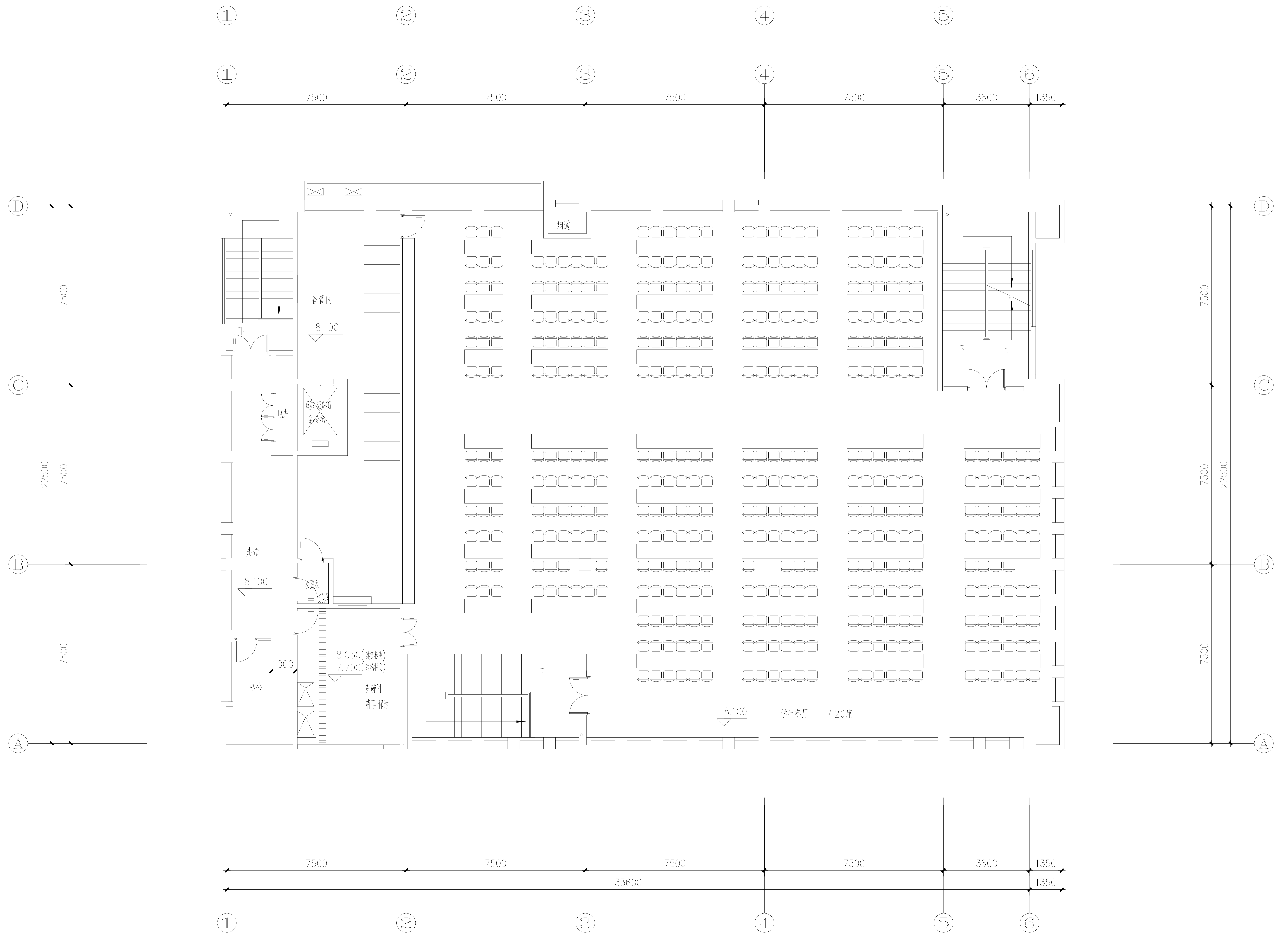
食堂三层平面图 1:100
