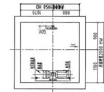
井道顶部平面图
