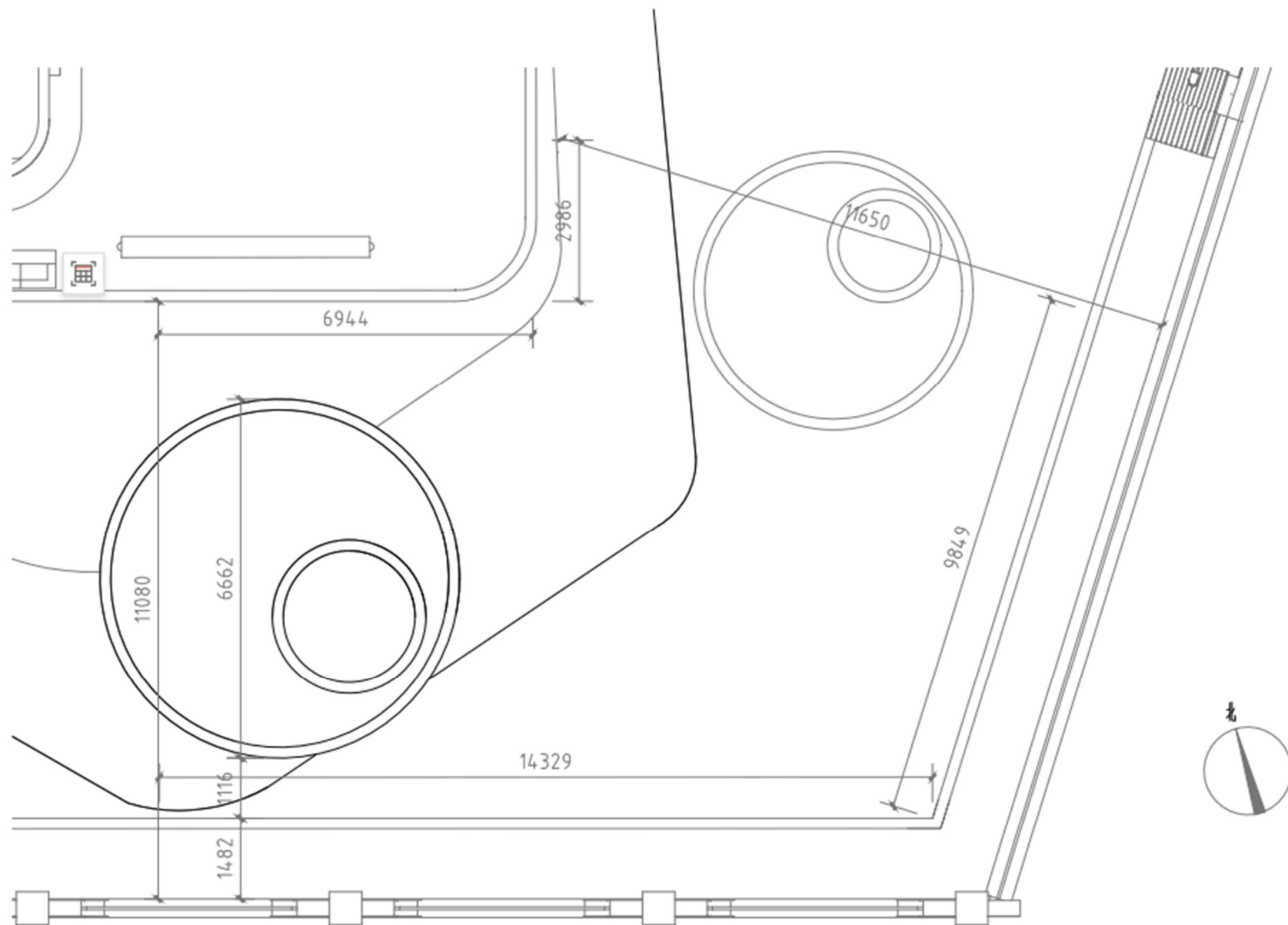
园特路幼儿园户外场地尺寸示意图
