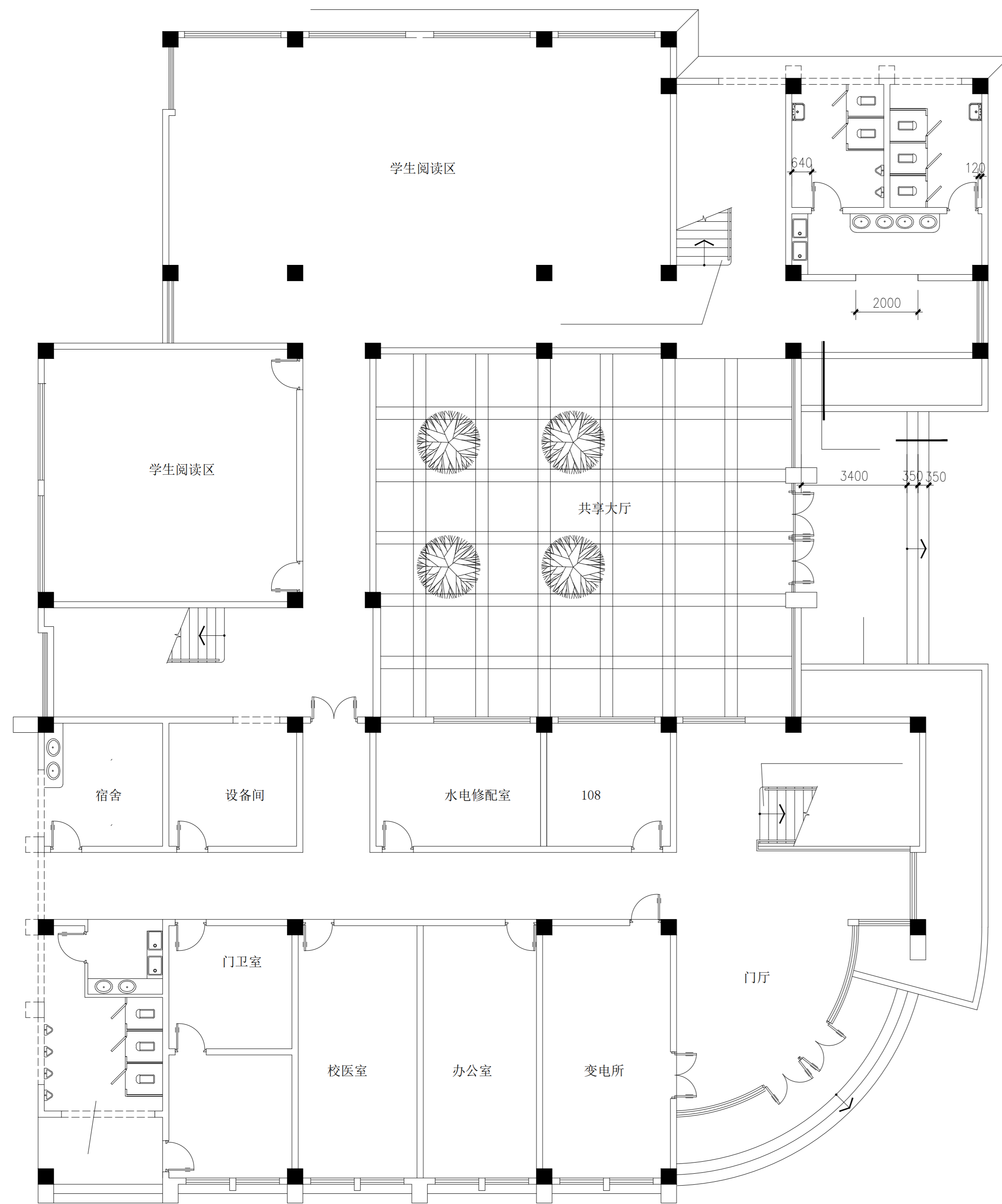
办公楼一层平面
