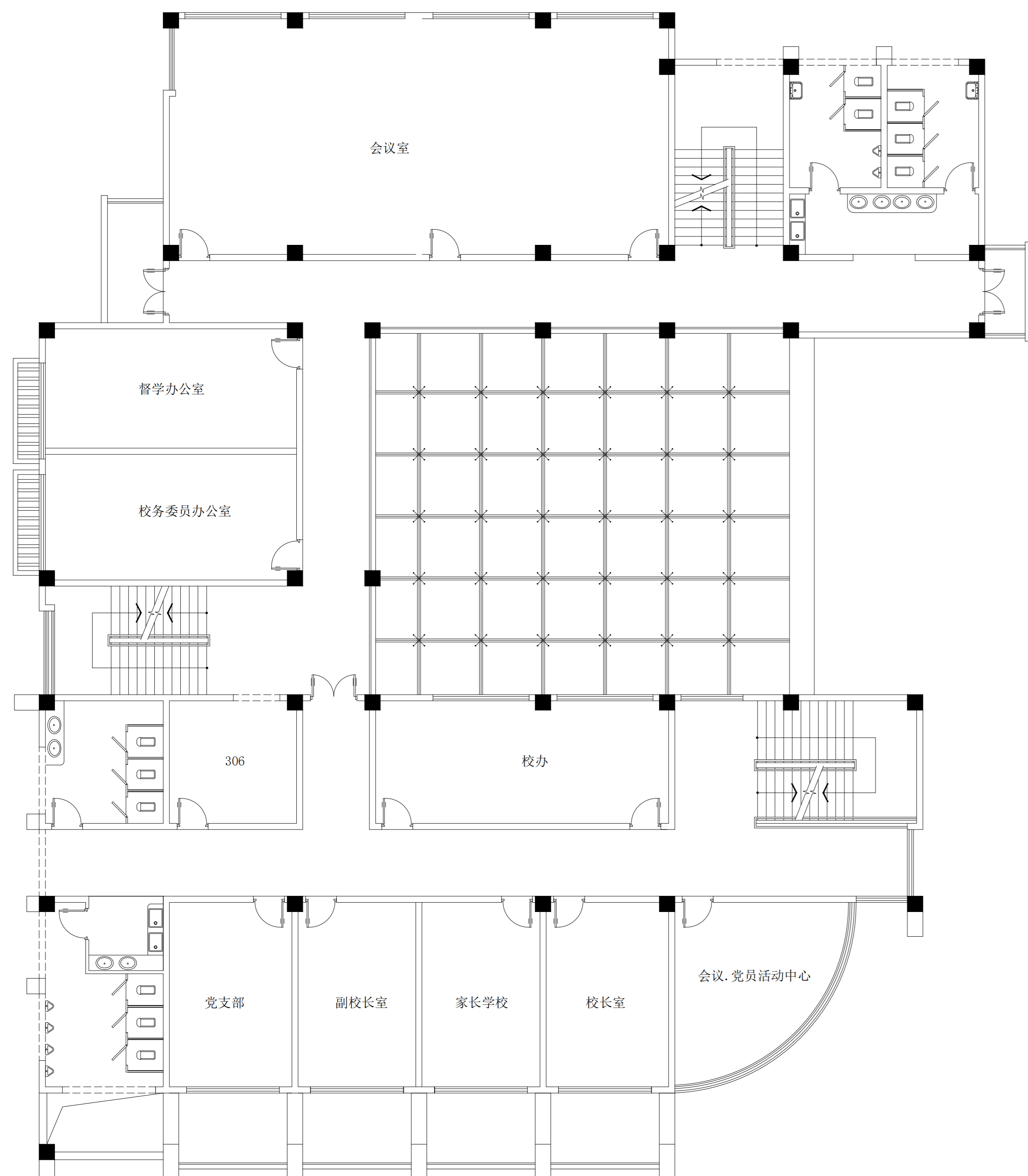
办公楼三层平面 1:100
