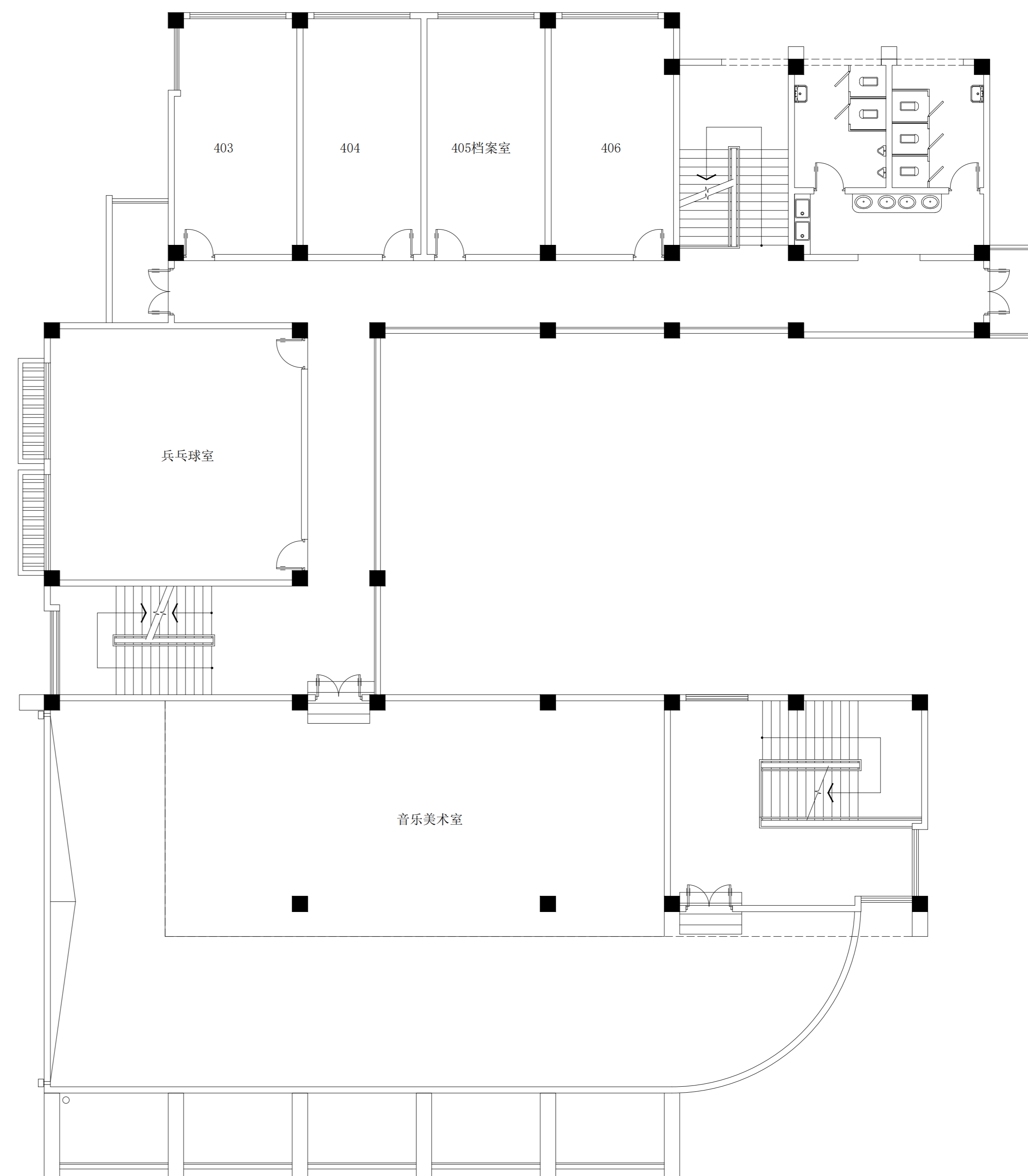
办公楼四层平面 1:100
