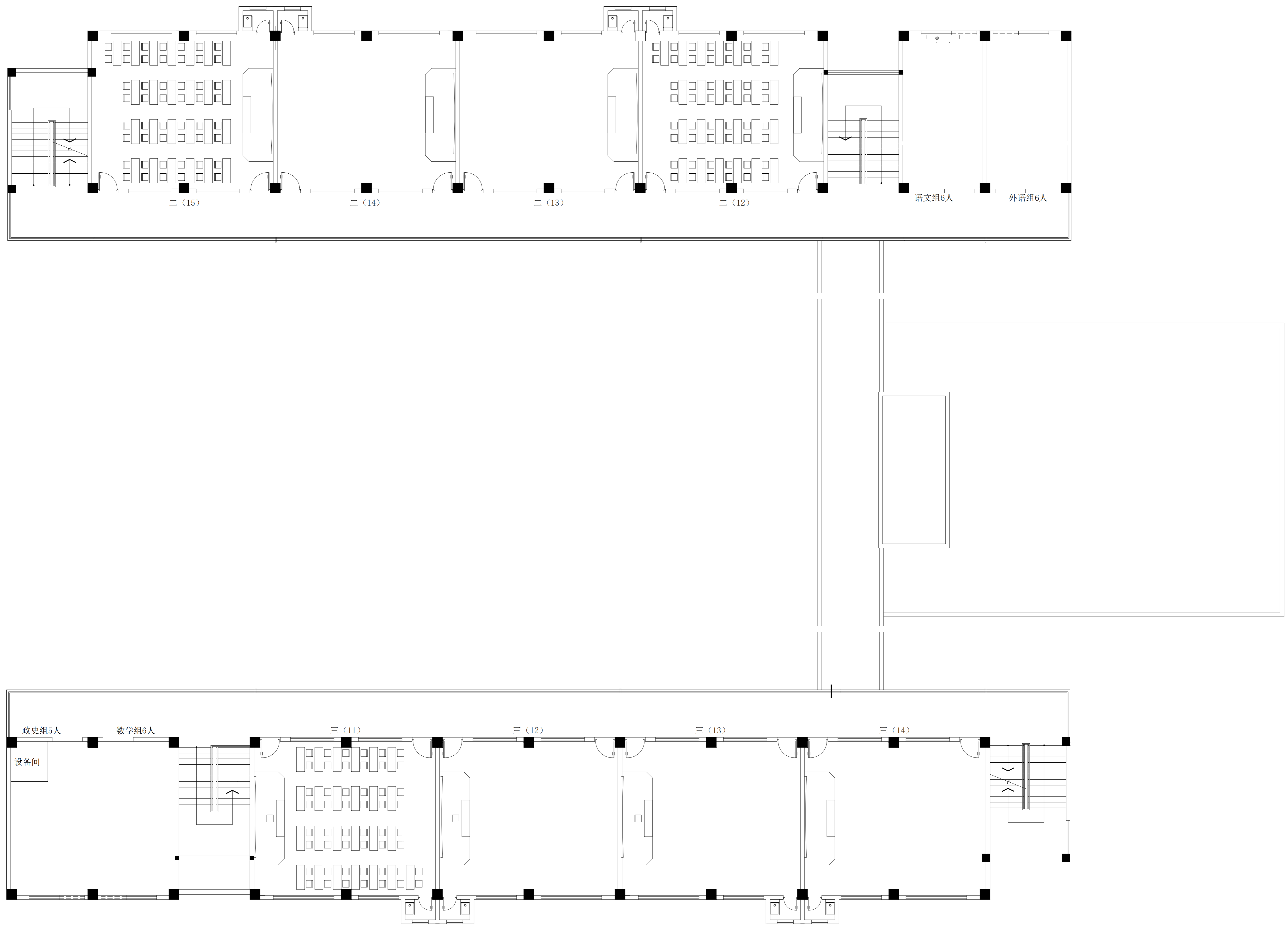
教学楼五层平面
