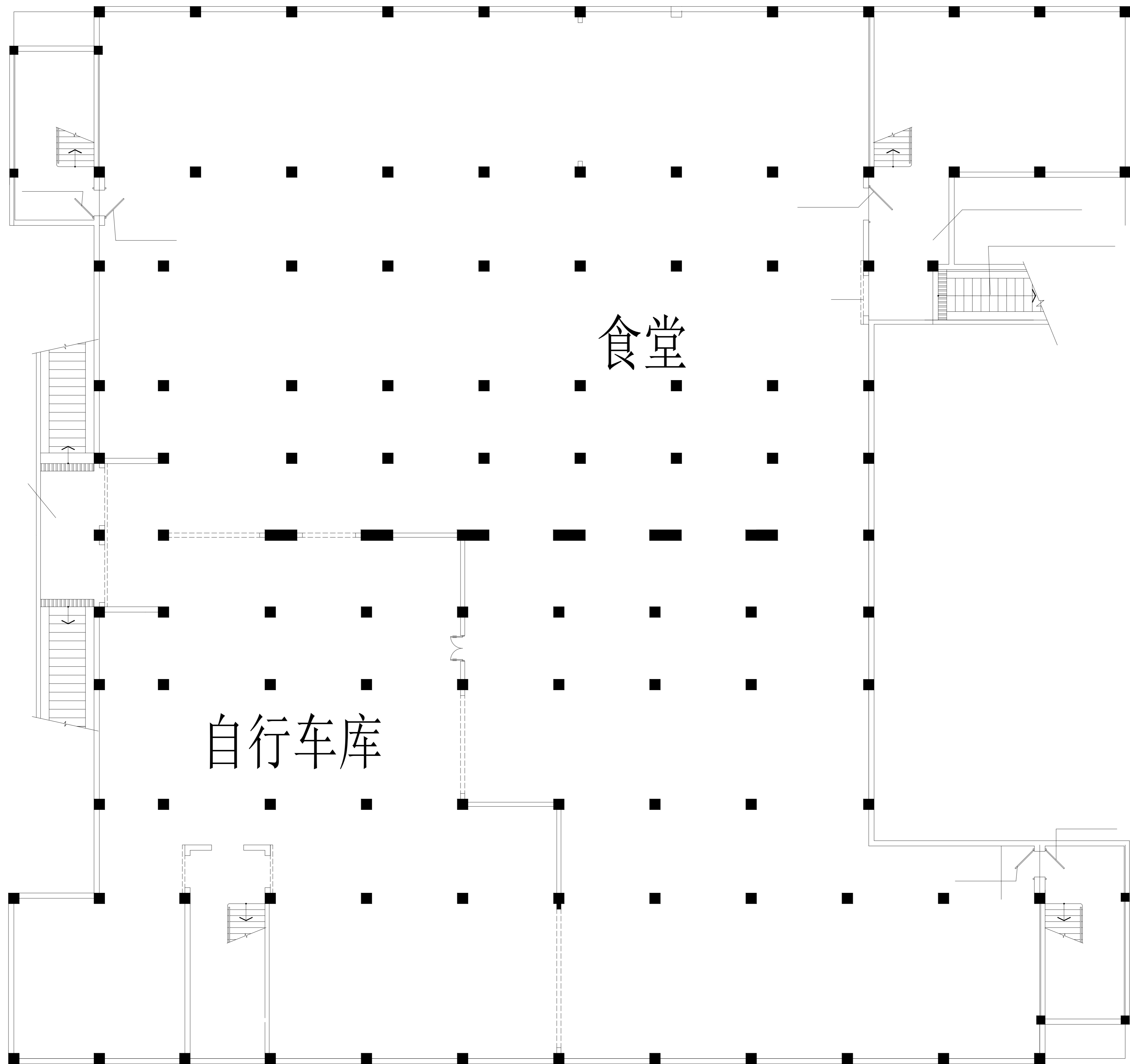
教学楼地下一层平面
