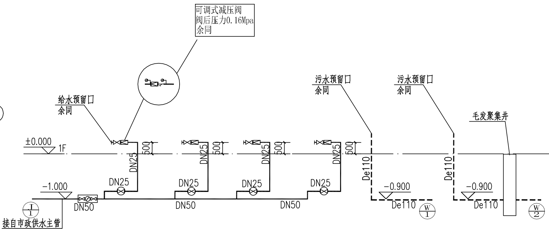
给排水管道原理图 1:100
