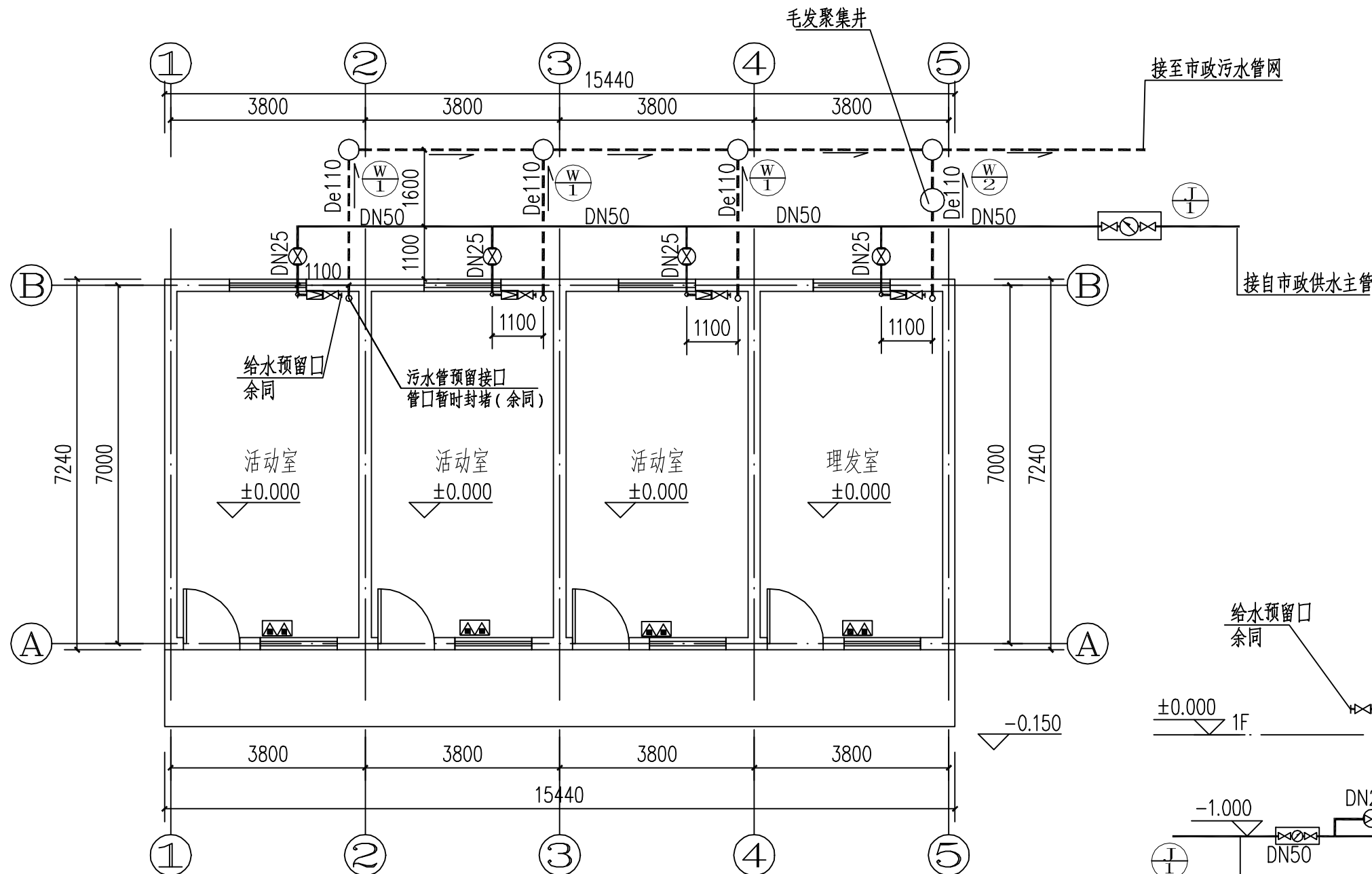
一层给排水平面图 1:100
